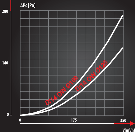
PERFORMANCE DE DÉBIT PRŮTOKOVÁ CHARAKTERISTIKA VÝKONNOSTI PRIETOKOVÁ CHARAKTERISTIKA VÝKONU
