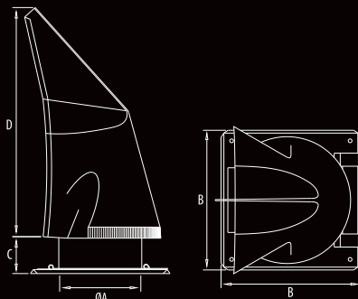
DIMENSION / ROZMĚRY / ROZMERY
