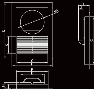
DIMENSION / ROZMĚRY / ROZMERY
