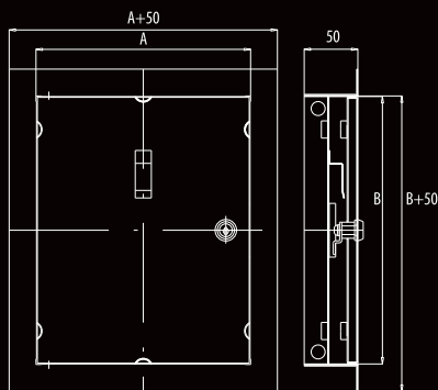
DIMENSION / ROZMĚRY / ROZMERY
